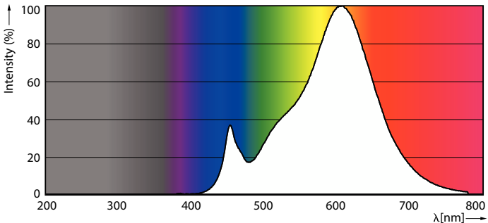
Spectral Power Distribution Colour - LEDStick 14W E27 DS FR DIM 1PF/6 AU
