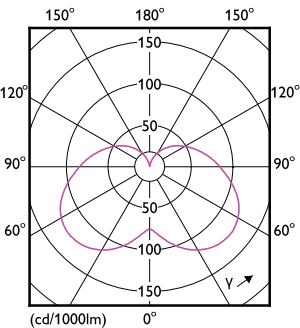
Light Distribution Diagram - LEDStick 14W E27 DS FR DIM 1PF/6 AU
