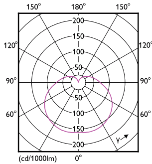
Light Distribution Diagram - LEDStick 10W E27 DS FR DIM 1PF/6 AU
