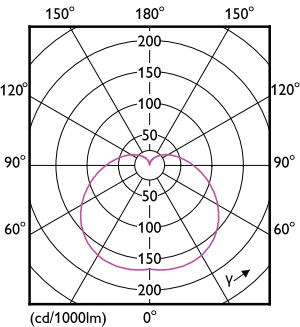
Light Distribution Diagram - LEDBulb 14W B22 DS FR DIM 1PF/6 AU
