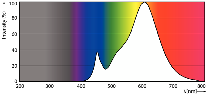
Spectral Power Distribution Colour - LEDBulb 14W B22 DS FR DIM 1PF/6 AU
