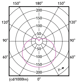
Light Distribution Diagram - LEDBulb 14W E27 DS FR DIM 1PF/6 AU
