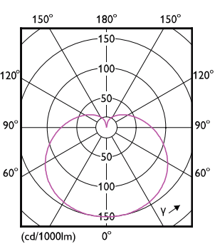
Light Distribution Diagram - LEDBulb 9W E27 DS FR DIM 1PF/6 AU
