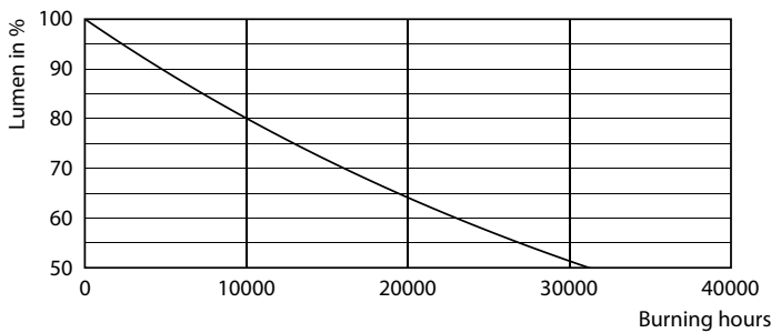
Lumen Maintenance Diagram - LEDSpot 35W DS ND MR16 12V 60D 1CT/6 AU
