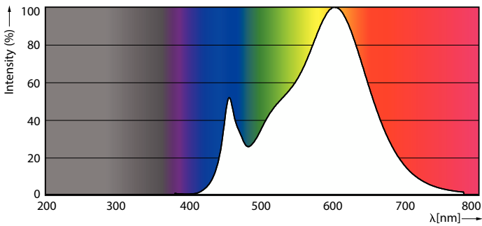
Spectral Power Distribution Colour - LEDBulb 8W B22 DS FR ND 1CT/6 AU
