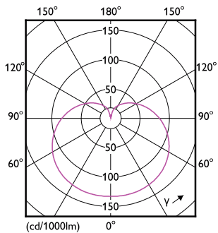
Light Distribution Diagram - LEDBulb 8W B22 DS FR ND 1CT/6 AU
