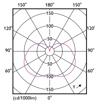
Light Distribution Diagram - LEDStick 6W B22 DS FR ND 1CT/6 AU
