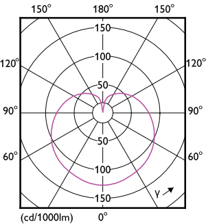
Light Distribution Diagram - LEDLuster 6W P45 6500K E27 ND FR AU 2CT
