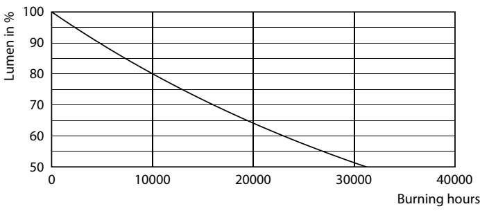
Lumen Maintenance Diagram - LEDLuster 6W P45 6500K E27 ND FR AU 2CT
