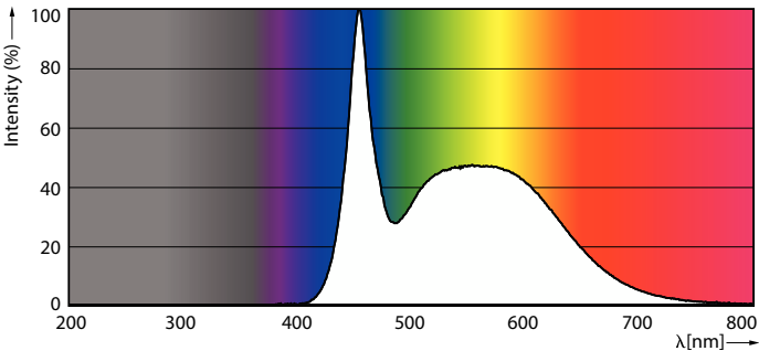
Spectral Power Distribution Colour - LEDLuster 6W P45 6500K E27 ND FR AU 2CT
