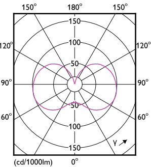
Light Distribution Diagram - LEDclassic 60W G93 2700K E27 D CL AU
