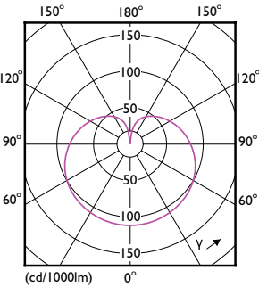
Light Distribution Diagram - LEDBulb 8W E27 965 230V 2PF/3 AU
