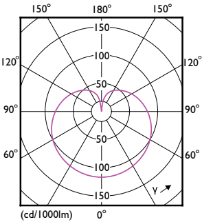
Light Distribution Diagram - LEDBulb 6W E27 930 230V 2PF/3 AU
