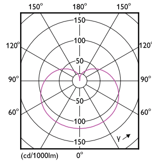
Light Distribution Diagram - 29A21/PER/850/FR/P/E26/D/HO 4/1PF
