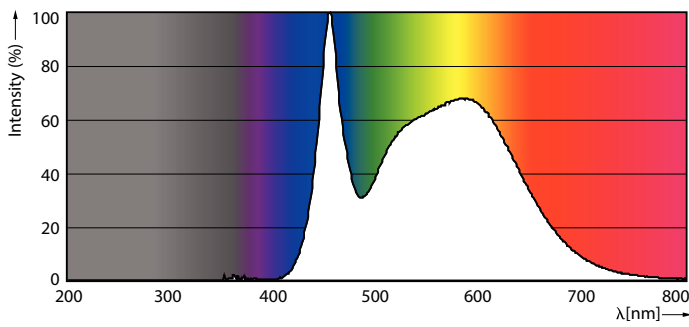
Spectral Power Distribution Colour - 9A19/LED/850/FR/P/ND 4/6FB
