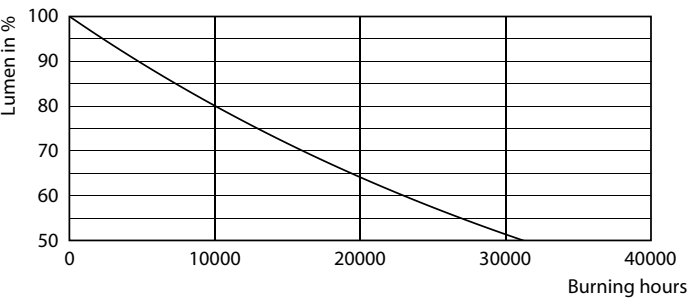
Lumen Maintenance Diagram - 4A19/PER/BUE/G/E26/ND 4/1PF
