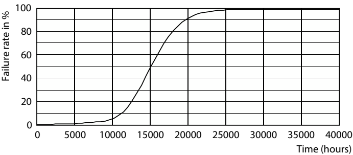
Life Expectancy Diagram - 4A19/PER/BUE/G/E26/ND 4/1PF
