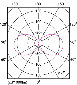
Light Distribution Diagram - 4A19/PER/BUE/G/E26/ND 4/1PF
