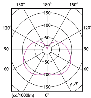
Light Distribution Diagram - LEDStick 9.5W E27 6500K 1PF/6 AU
