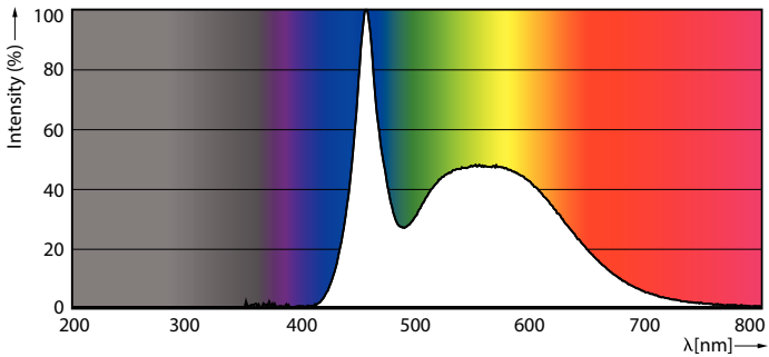
Spectral Power Distribution Colour - LEDStick 9.5W E27 6500K 1PF/6 AU
