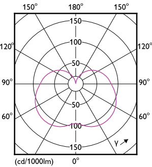
Light Distribution Diagram - LEDStick 9.5W E27 6500K 1PF/6 AU
