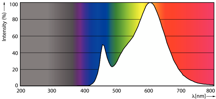
Spectral Power Distribution Colour - LEDStick 9.5W E27 3000K 1PF/6 AU
