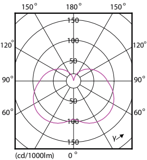
Light Distribution Diagram - LEDStick 9.5W E27 3000K 1PF/6 AU
