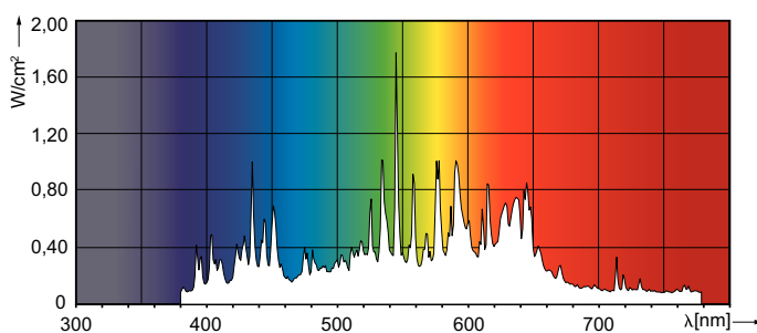
Spectral Power Distribution Colour - MASTERCouleur CDM-T MW eco 360W/842 E40
