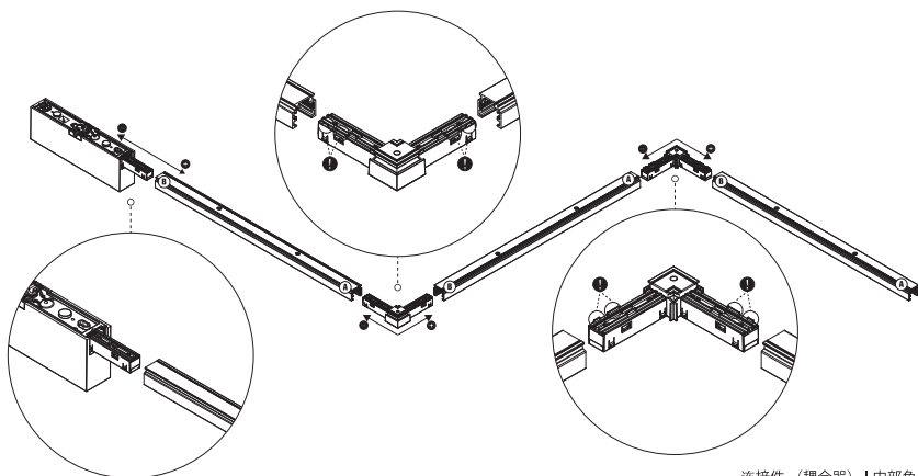
连接件（耦合器）| 内部角 Corner connector internal
