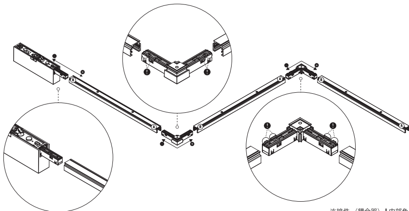
连接件（耦合器）| 内部角 Corner connector internal
