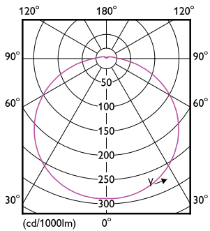
Light Distribution Diagram - 26UFO/PER/850/FR/P/E26/ND 4/1PF
