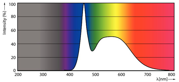
Spectral Power Distribution Colour - 26UFO/PER/850/FR/P/E26/ND 4/1PF
